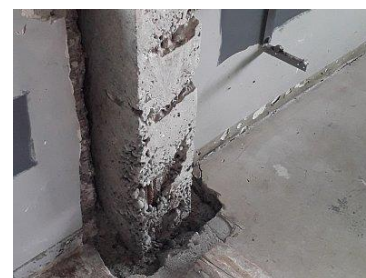
Sanierung/Umbau Geschäftshaus
